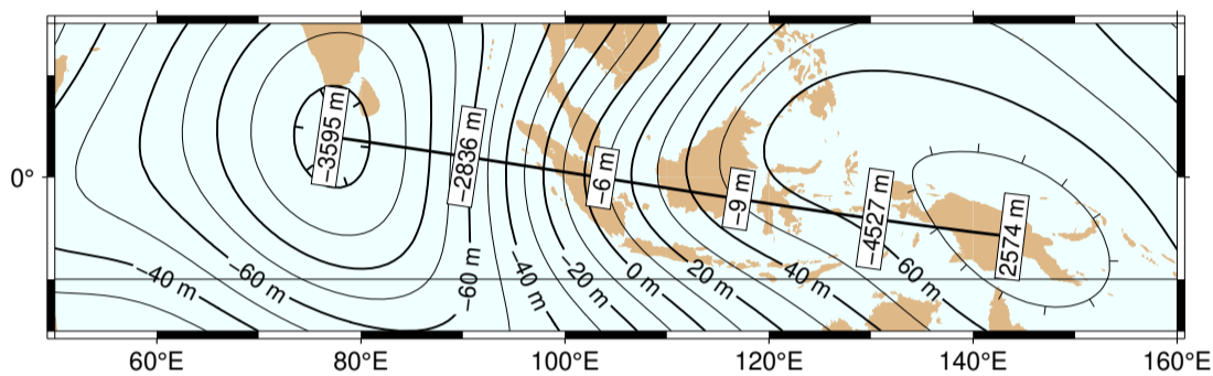
图 8: 标注的位置和内容来自不同的数据集
