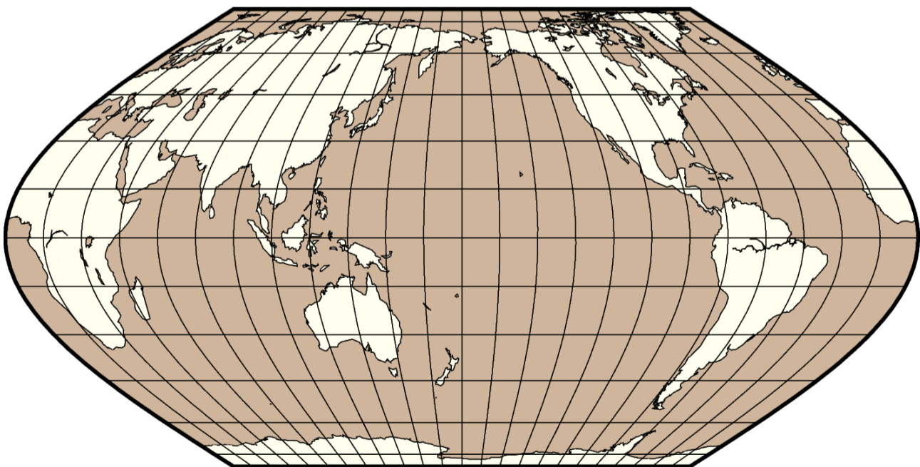
图 23: Eckert VI 投影绘制全球图
