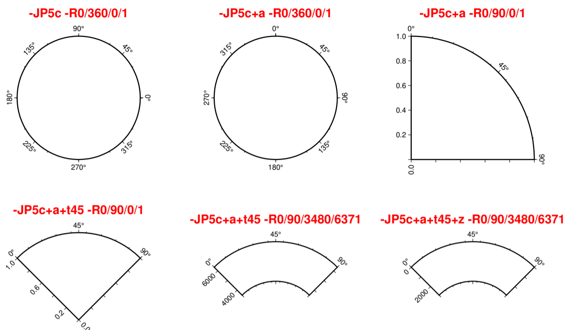
图 6: 极坐标用法示例
