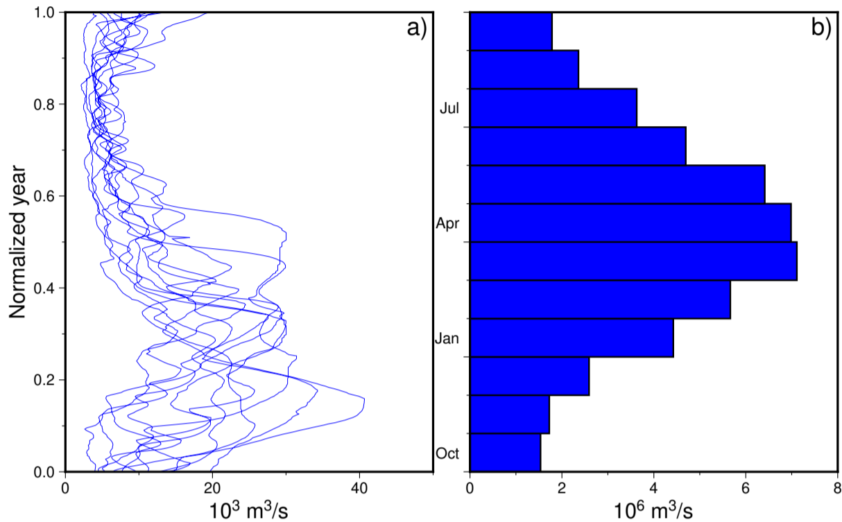
图 22: a) 归一化后一年内的密西西比河日流量, b) 10 年的密西西比河月流量, 以 9 月为起点
