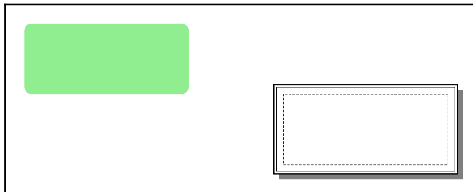
图 10: GMT 修饰物背景面板
