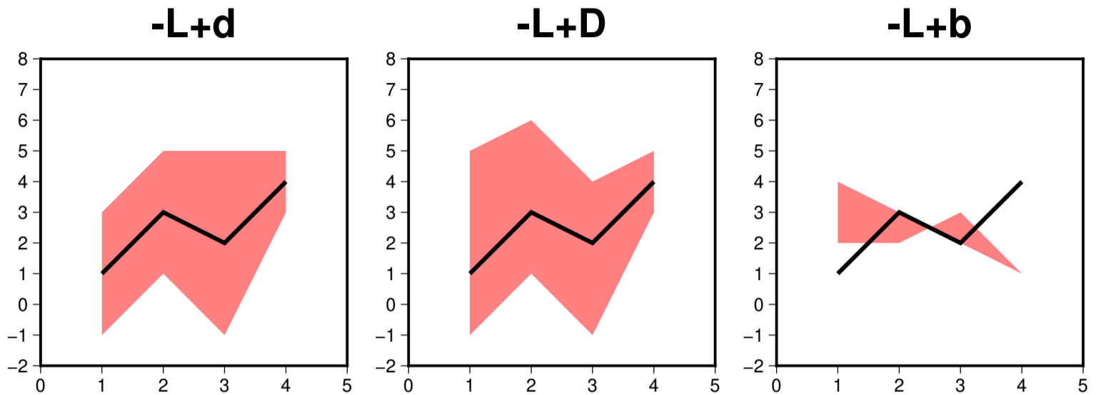
图 9: 围绕线条的包络
