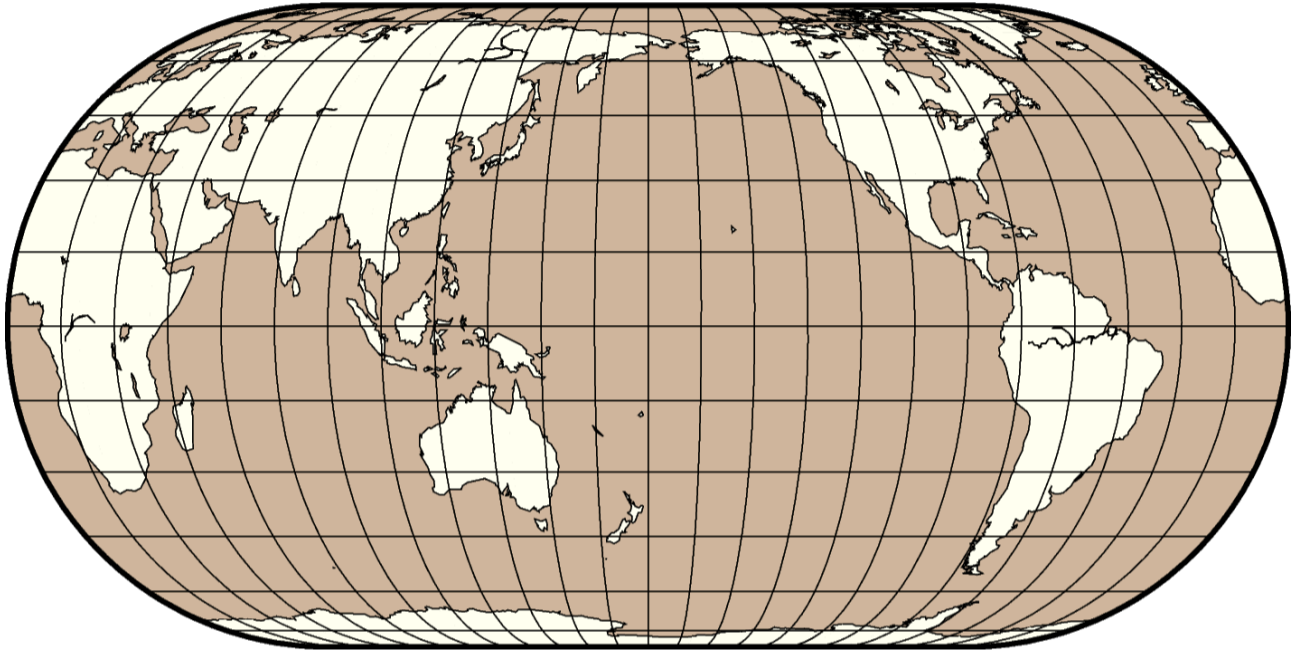
图 22: Eckert IV 投影绘制全球图
