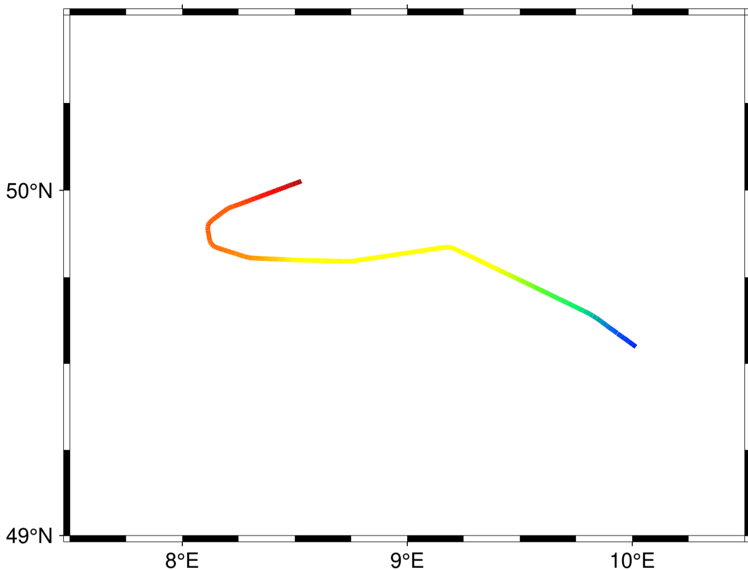
图 3: 绘制颜色渐变的线段
