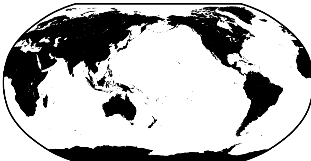
图 1: GSHHG: 全球高分辨率海岸线数据
