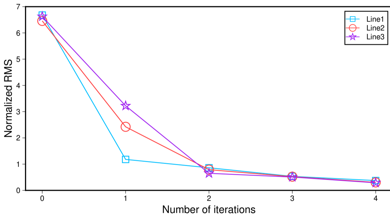
图 1: 绘制点线图及其图例
