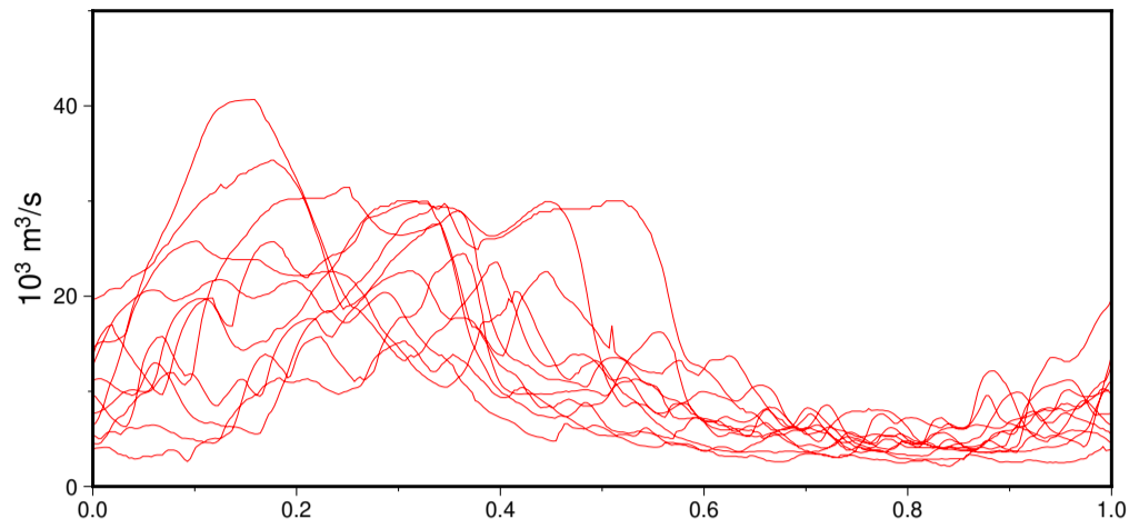
图 20: 归一化年份下的密西西比河日流量时间序列图
