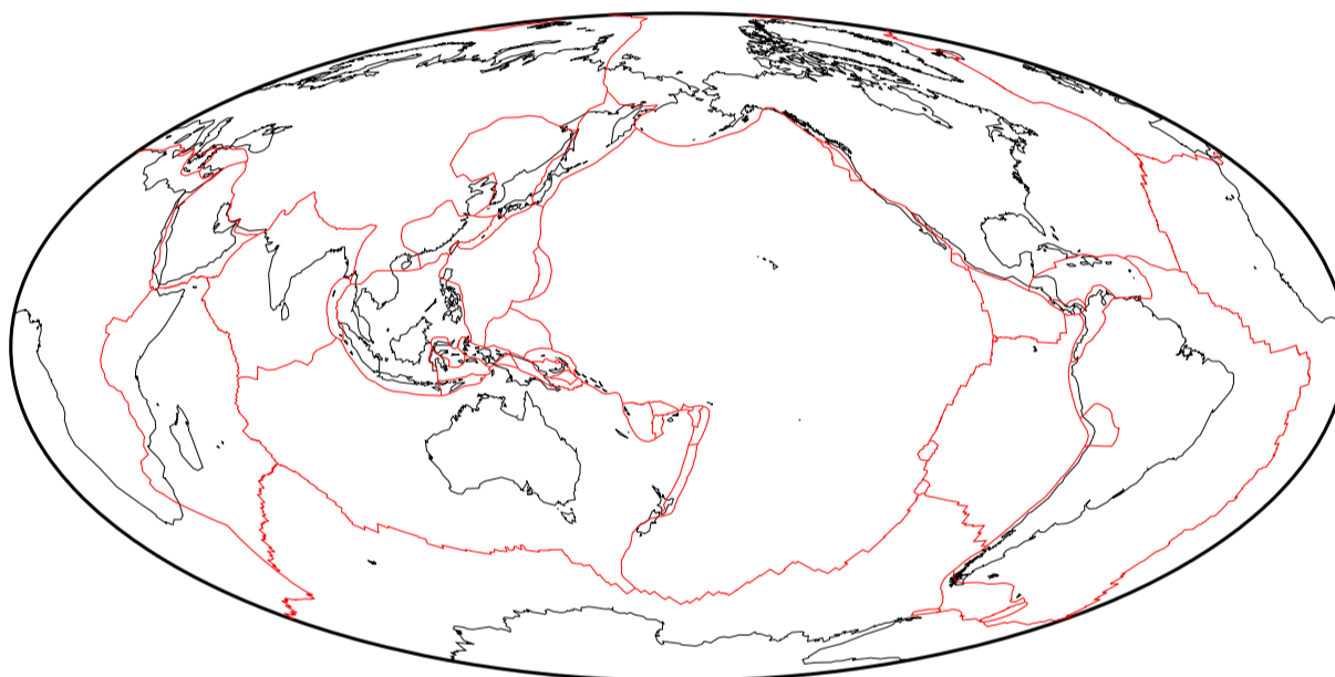
图 3: PB2002 全球板块边界
