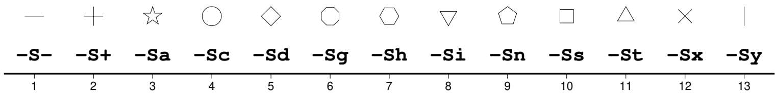
图 11: plot -S 选项示意图
